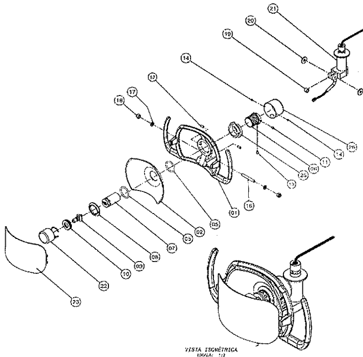
VISTA ISOMÉTRICA ESCALA: 1:2
