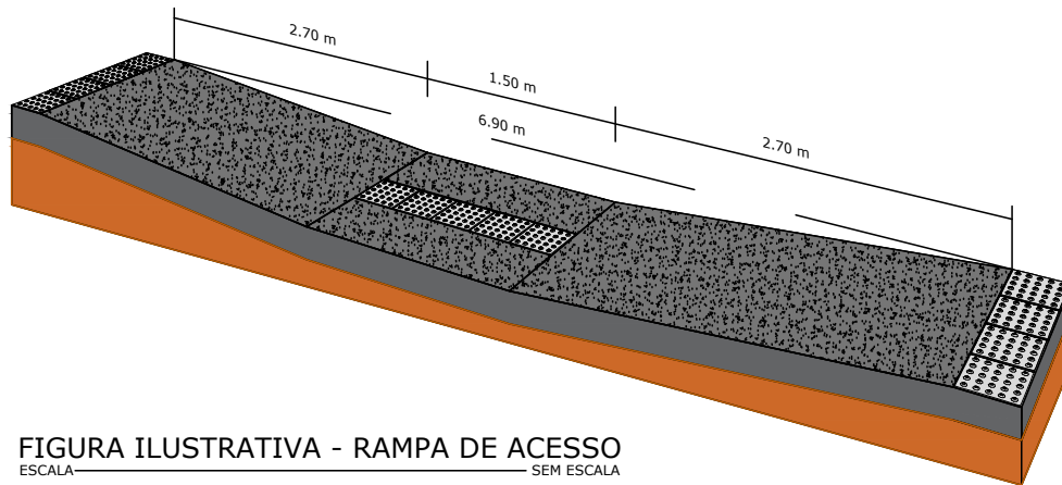
DETALHE DO ACESSO À RAMPA SEM ESCALA
