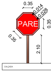
PLACA DE SINALIZAÇÃO SEM ESCALA
