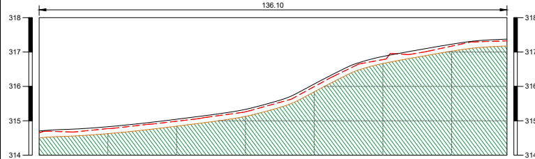
Perfil Longitudinal Escala: H.....1/5.000 V.....1/500
