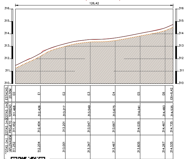
Perfil Longitudinal Escala: H.....1/5.000 V.....1/500
